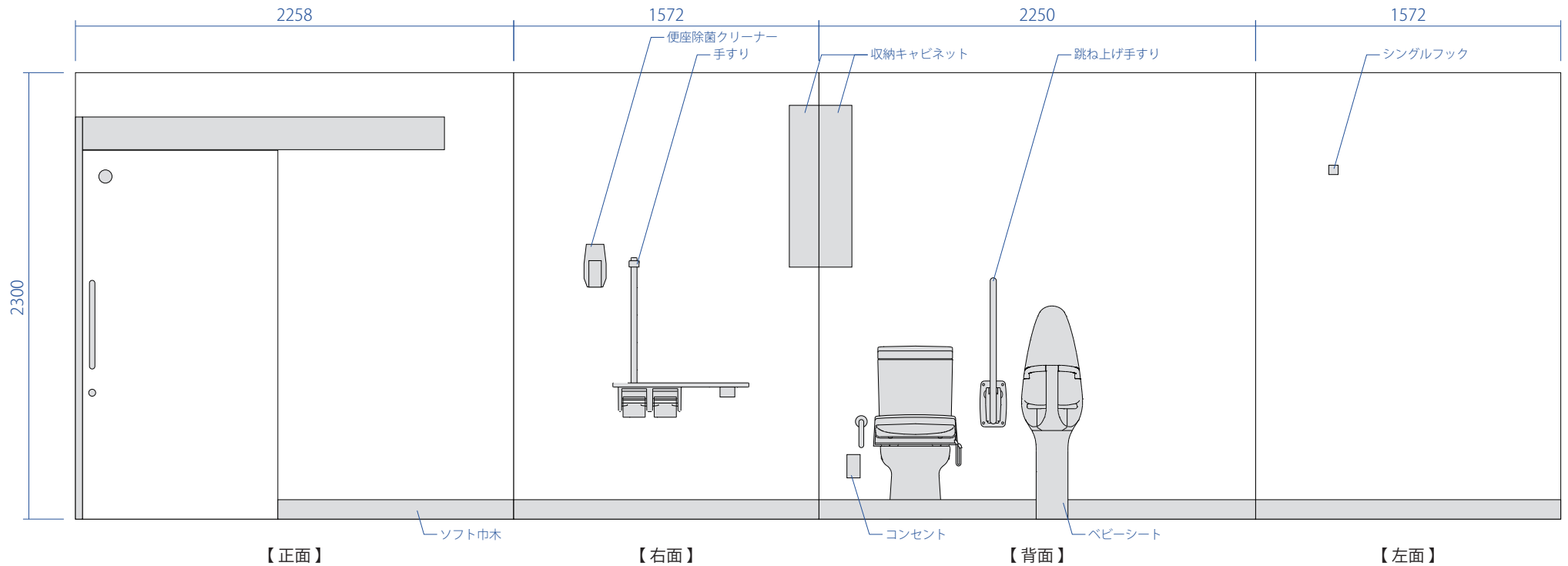
【個室内展開図】
